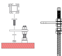
Kit de fixation toiture tôle ondulée
